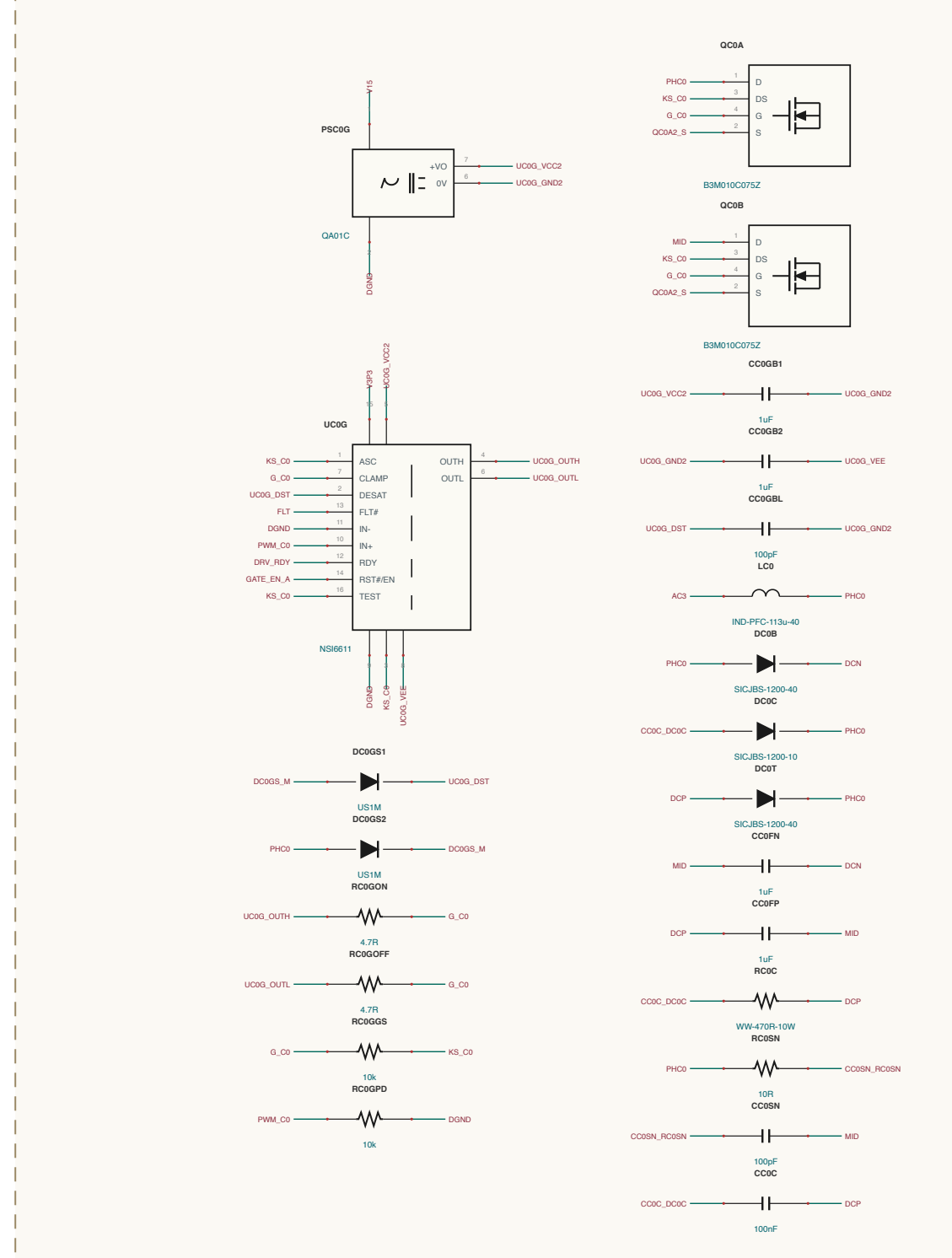
VIENNA-PFC / PHASE-C0
