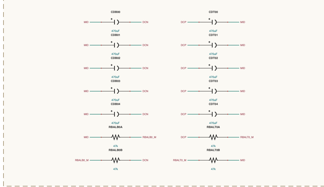
DC-LINK / LINK-BANK-0
