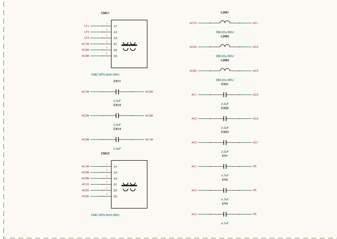
INPUT-EM / EMI-FILTER
