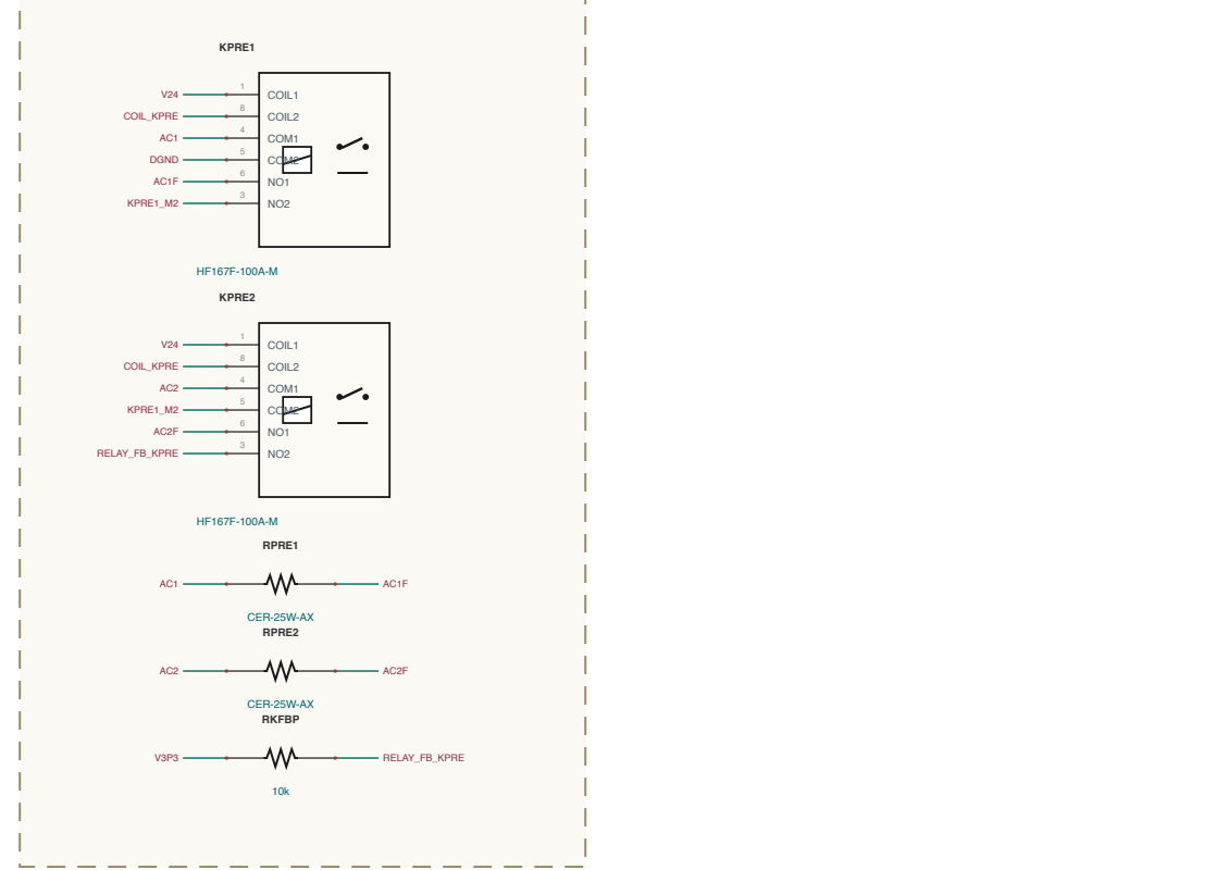
INPUT-EM / PRECHARGE
